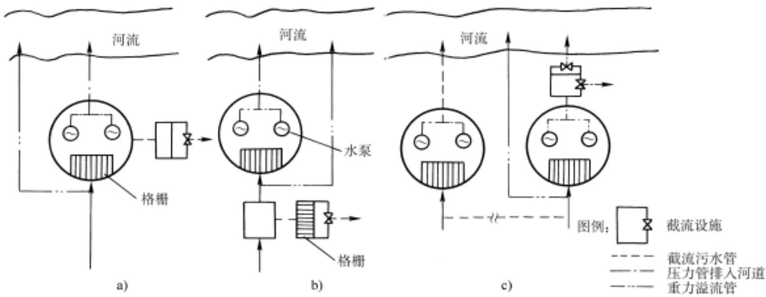
图 1—6 泵前截泵站的形式 a) G_1 型 b) G_2 型 c) G_3 型
