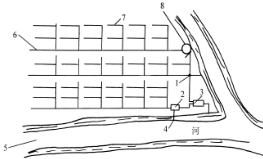
图 1—2 截流式合流制排水系统示意图
