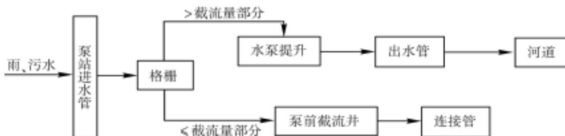
图 1—9 降雨期间的雨水、污水流程图
