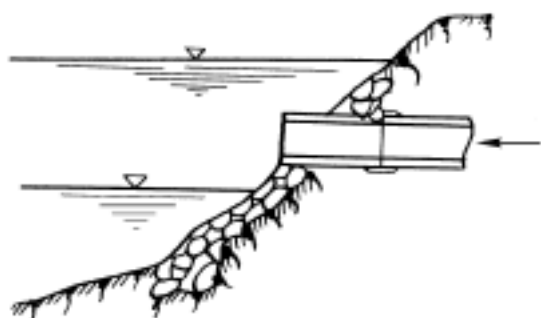
图 1—4 护坡式出水口
