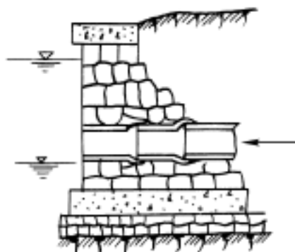
图 1—5 挡土墙式出水口
