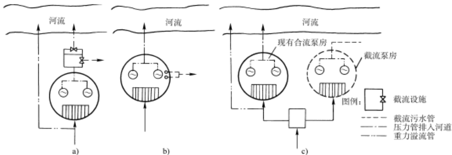
图 1—7 泵后截泵站的形式
