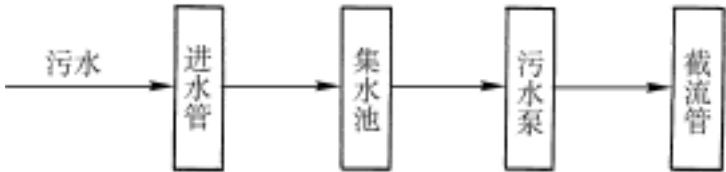
图 1—10 旱流期间污水流程图
