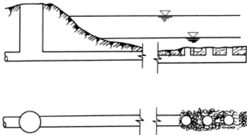
图 1—3 伸入江河的分散式出水口
