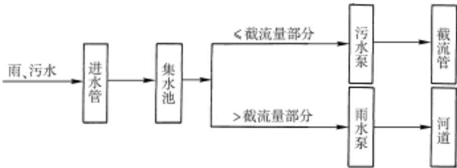
图 1—11 降雨期间的雨水、污水流程图
