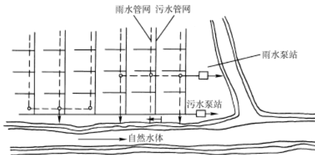
图 1—1 分流制排水系统示意图
