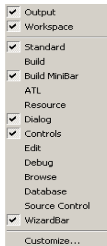
图 1.15 快捷菜单
