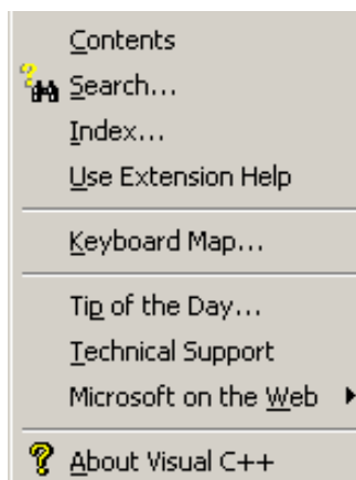
图 1.10 Help 菜单
