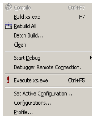
图 1.7 Build 菜单
