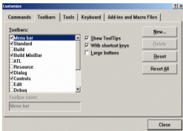
图 1.14 “Customize”对话框
