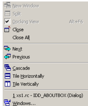
图 1.9 Window 菜单
