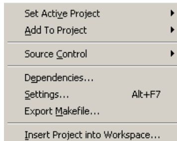
图 1.6 Project 菜单
