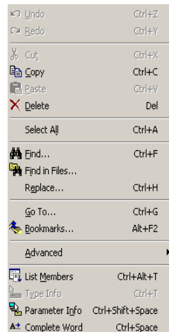
图 1.3 Edit 菜单
