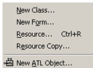
图 1.5 Insert 菜单
