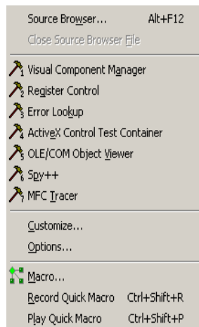
图 1.8 Tools 菜单
