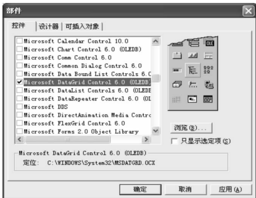
图 1-9 “部件”对话框
