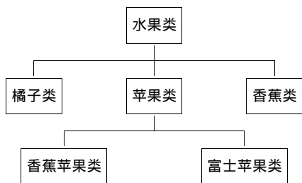
图 15-2 类继承关系
