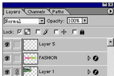
图 4-4 合并链接层
