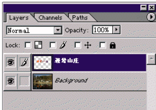
图 2-3 建立链接层
