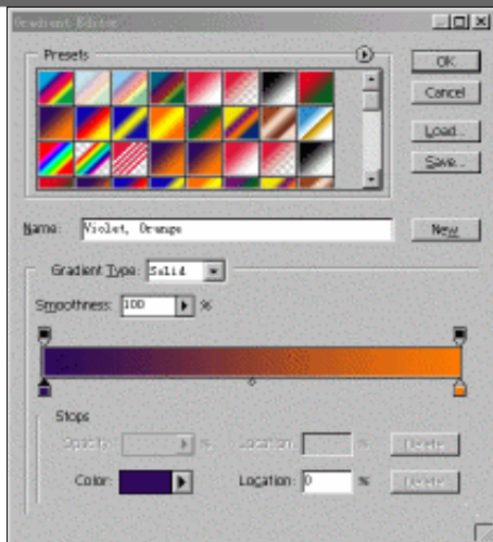
图 1-2 渐变编辑器
