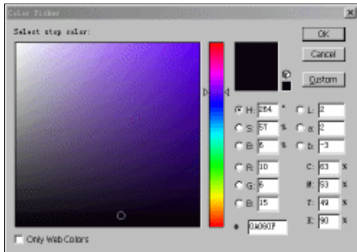
图 1-3 采色板
