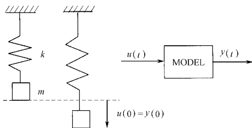
图 1-11 例 1-1 的谐振系统及其模型
