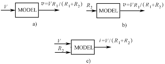
图 员源 图 员源所示系统的模型
