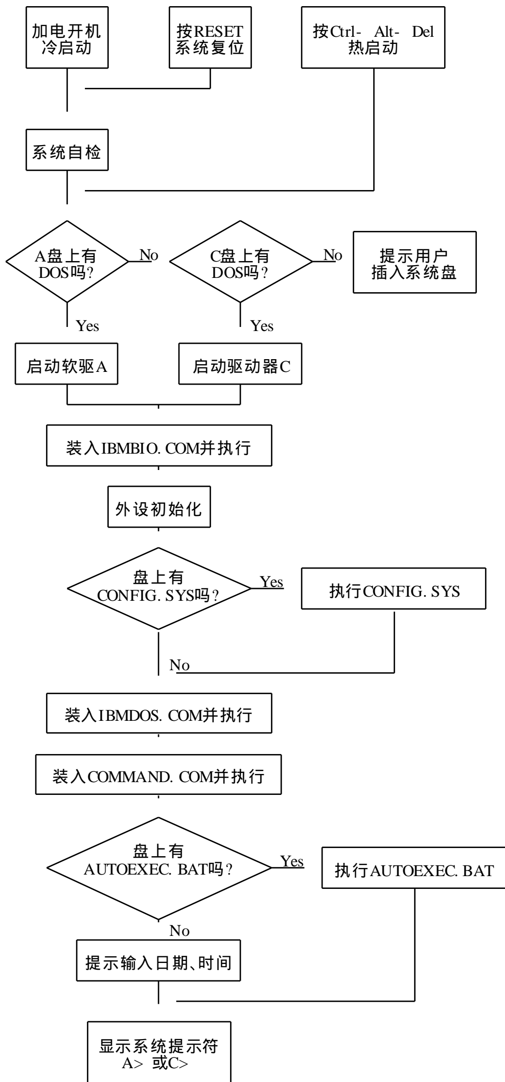
图 1.1 DOS 系统启动过程
