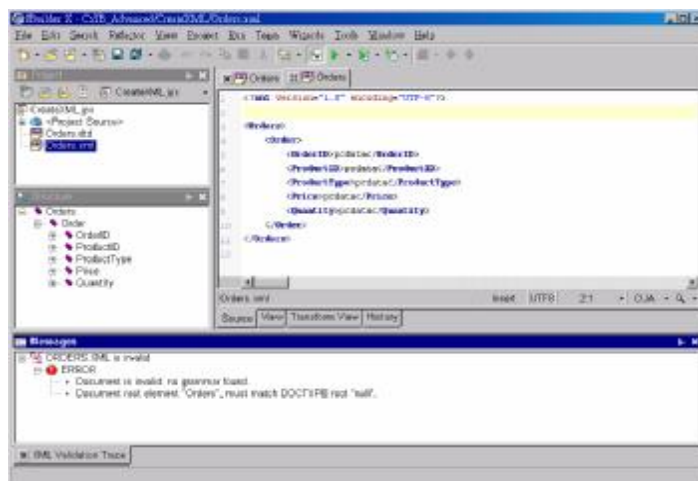
图 1-8 缺少 DOCTYPE 声明，无法进行检核程序
