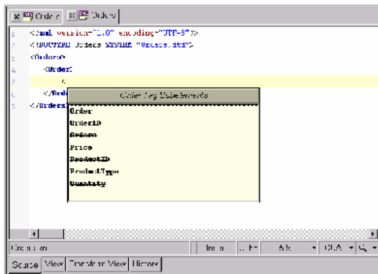
图 1-4 XML TagInsight 功能
