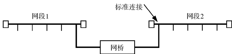
图 1 源原 两个网络通过网桥实施连接的示意图
