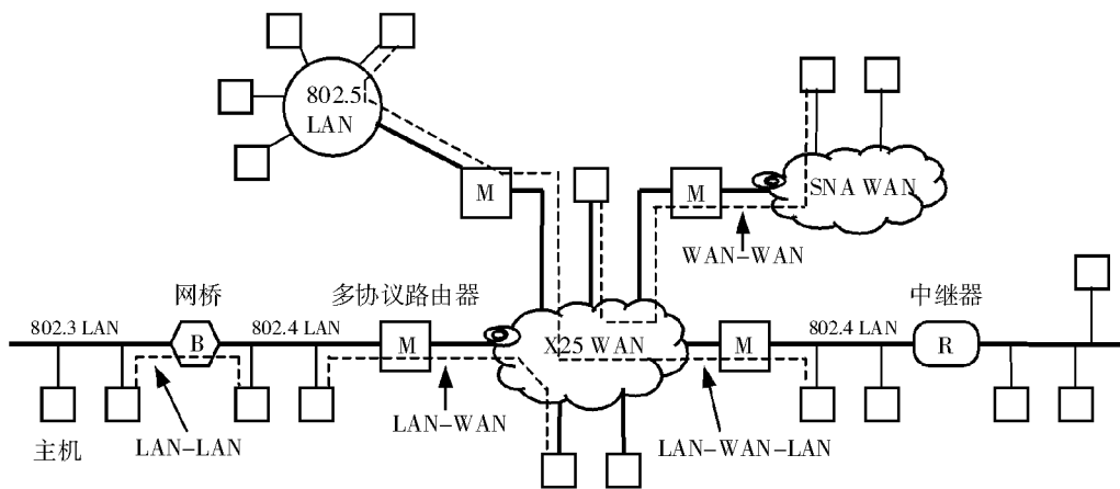
图 1-1 网络互联方式示意图
