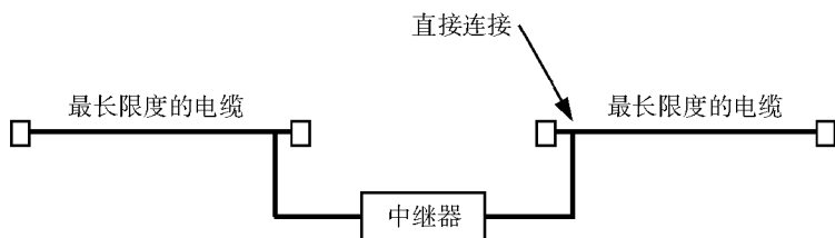
图 4-1-1 用中继器连接两条电缆扩展的局域网
