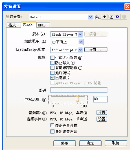
图 1-6 Flash 选项卡
