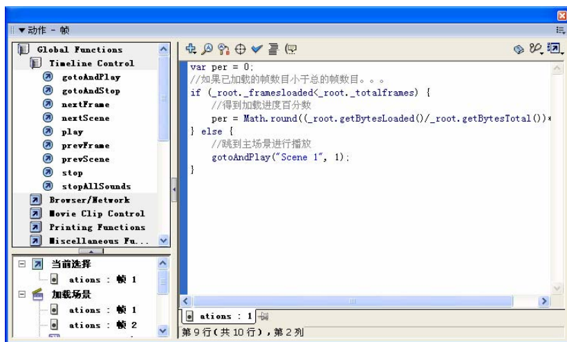
图 1-18 “动作”面板
