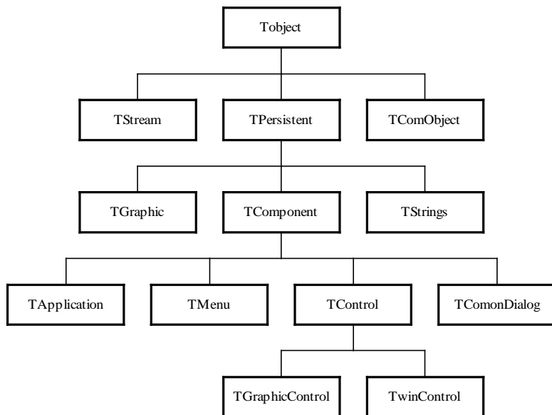
图1-1 VCL中主要的类之间的层次关系
