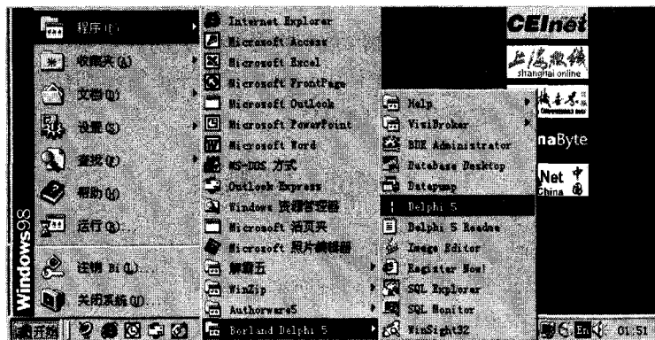
图 1.14 运行 Delphi 5
