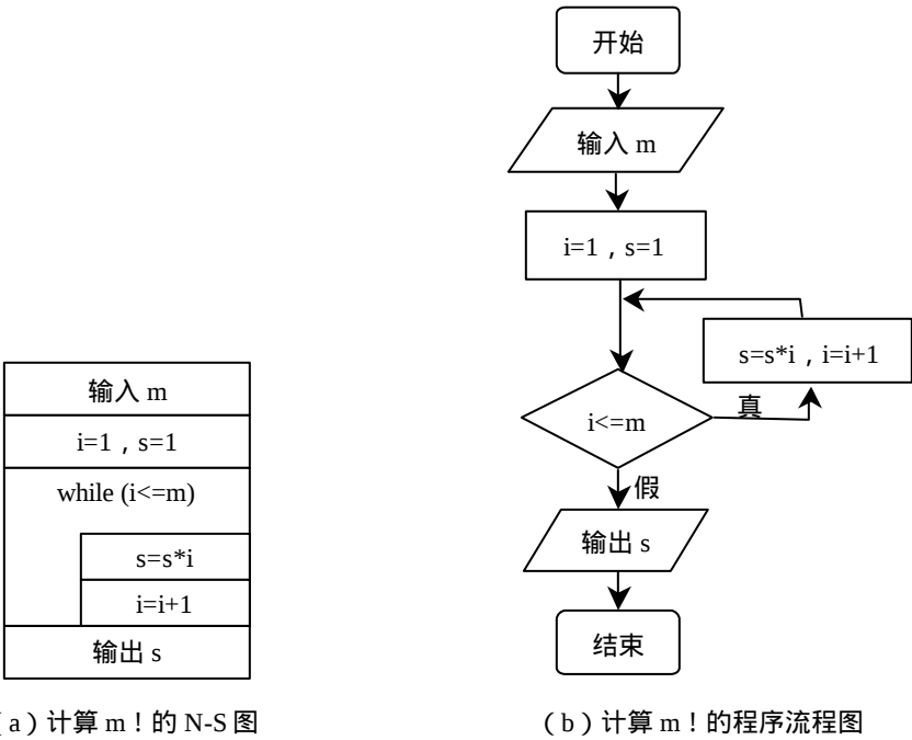
图 1.2 计算 m! 的 N-S 图和程序流程图
