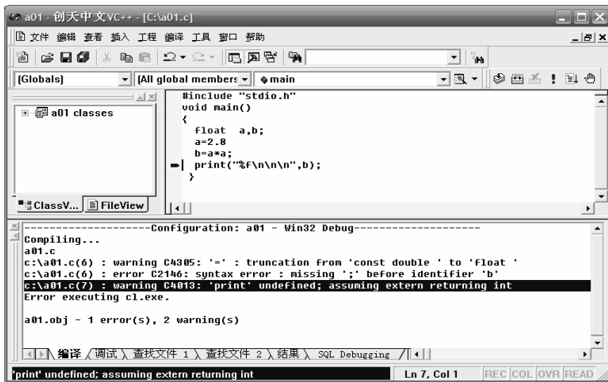
图 1-7 错误定位
