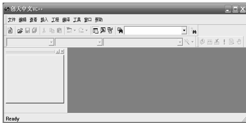
图 1-2 VC++ 6.0 界面
