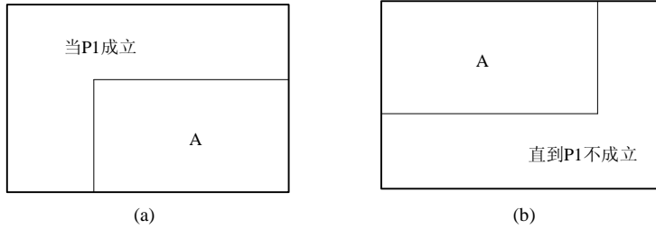
图 1.6 循环结构
