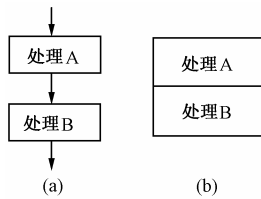
图 1.2 顺序结构
