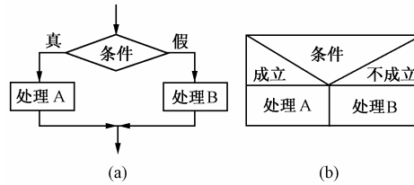
图 1.3 分支结构
