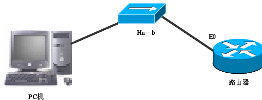
图 1-9 实验 2 的设备连接
