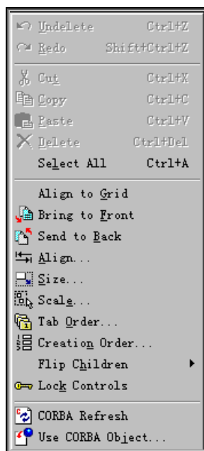
图 1-6 Edit 菜单
