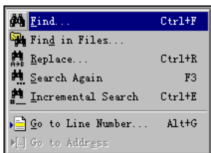
图 1-11 Search 菜单
