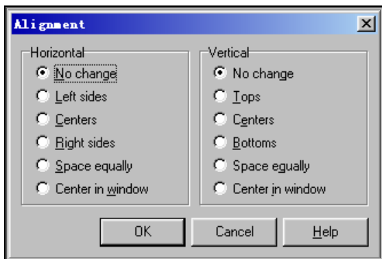
图 1-7 Alignment 对话框
