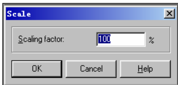
图 1-9 Scale 对话框
