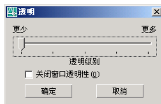
图 1-9 “透明”对话框
