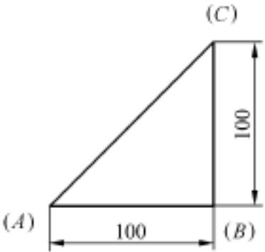
图 1-16 三角形
