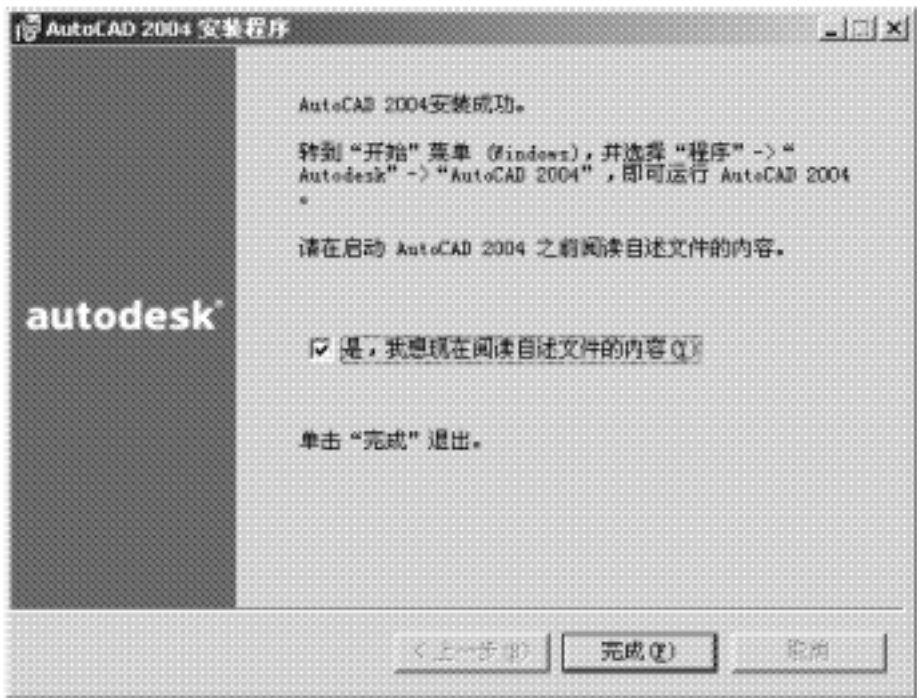
图 1 - 7 安装成功
