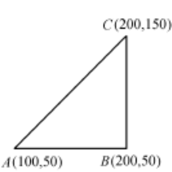
图 1-15 三角形
