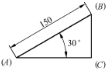
图 1-17 三角形
