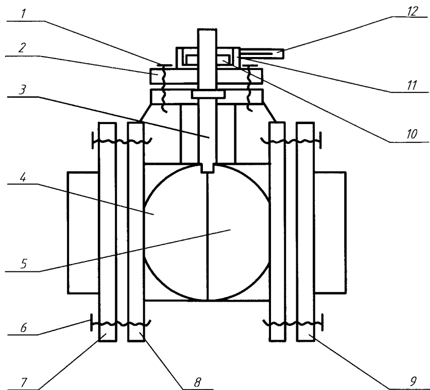
球阀装配示意图
