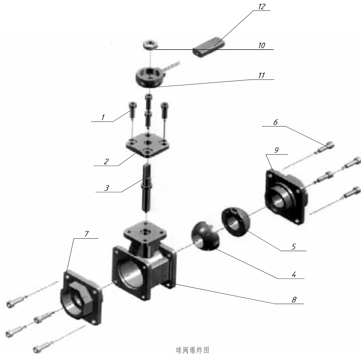
球阀爆炸图
