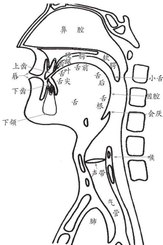
图1 发音器官 (摘自胡壮麟主编《语言学教程》第五版)
