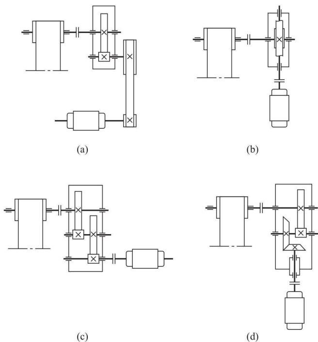
图 2-1 带式输送机的传动方案
