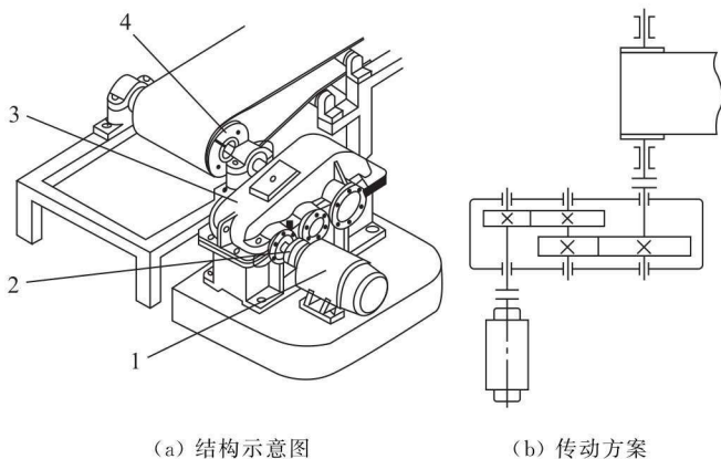
图 1-1 带式输送机的传动装置
