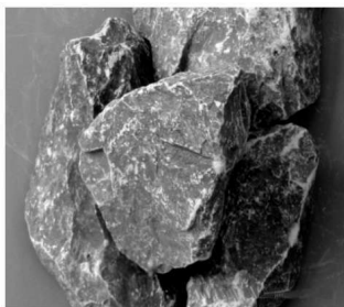
图 1.1 石灰岩
