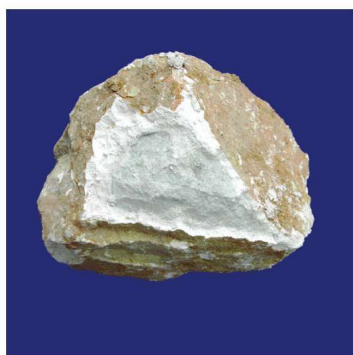
图 1.4 欠火石灰
