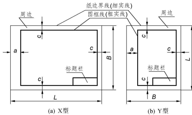
图 1-2 留装订边的图纸格式
