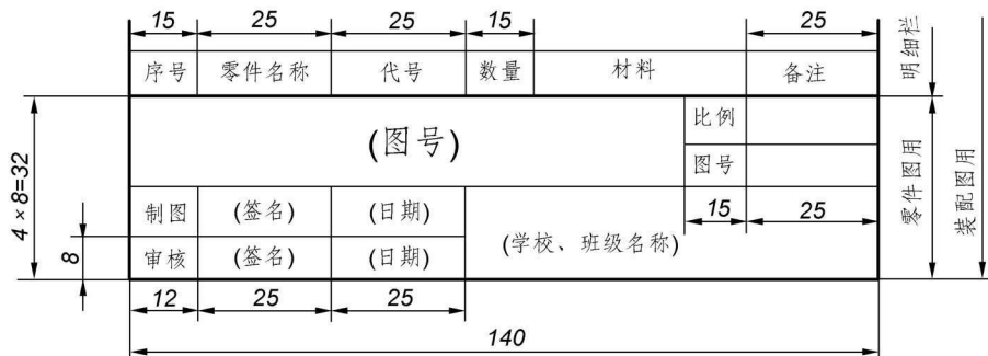
图 1-4 标题栏及明细栏格式
