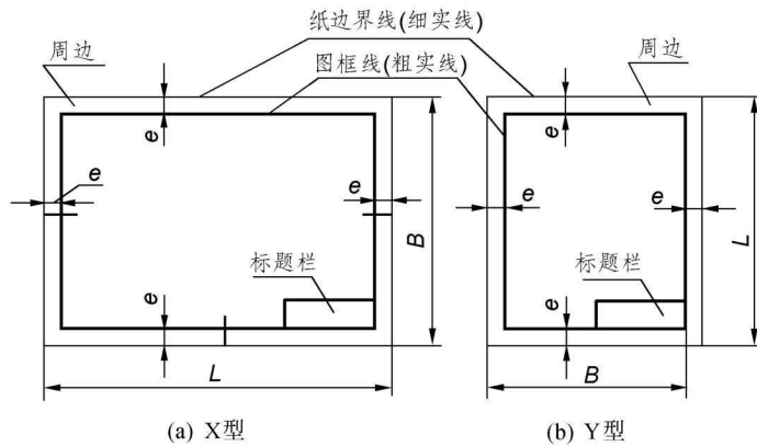
图 1-3 不留装订边的图纸格式
