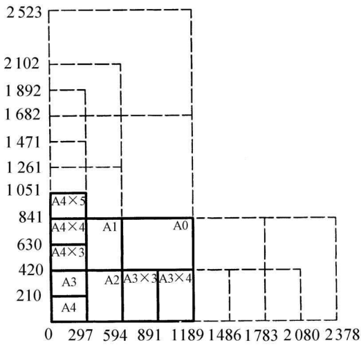
图 1-1 图幅尺寸及加长
