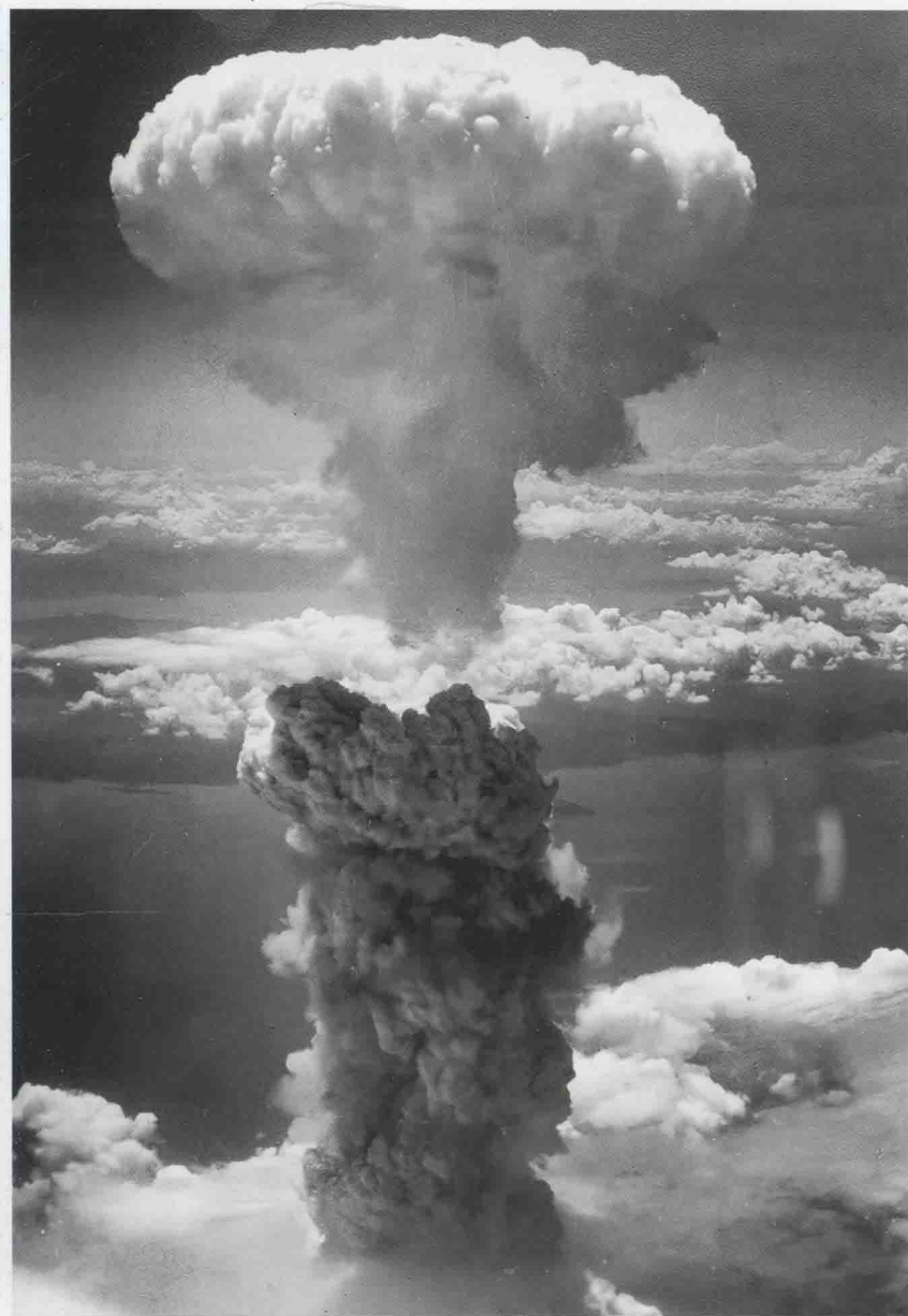
核弹爆炸
