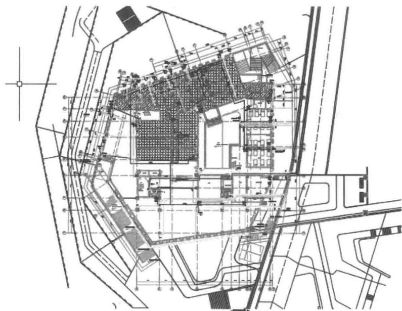
图 2.1-8 图层冻结前
