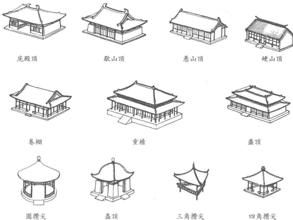
中国古代建筑屋顶形式图
