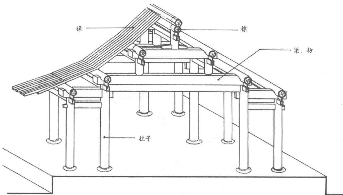
中国古代建筑木构架示意图
