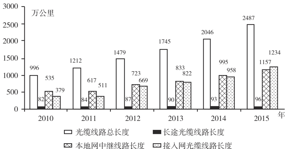
2010—2015年各种光缆线路长度对比情况
