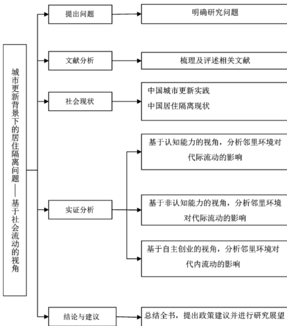
图 1-3 研究框架图
