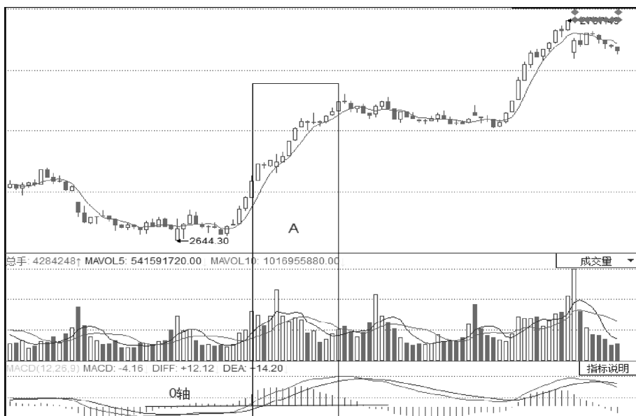
图 1-2 上证指数 15 分钟 K 线图
