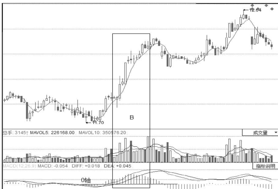
图 1-3 白云机场 15 分钟 K 线图
