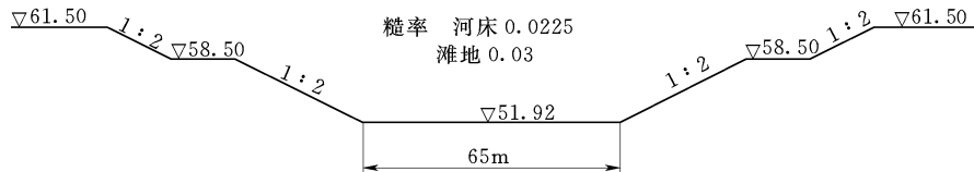
河道断面图
