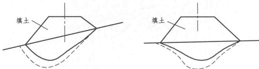
图 1-5 地基的应力分布及塑性变化趋势 [3]
