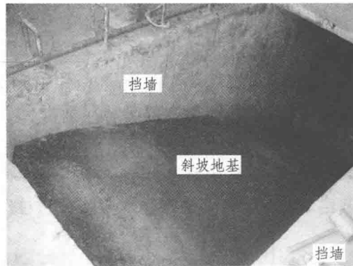
图 1-8 室内模型试验槽 [39]
