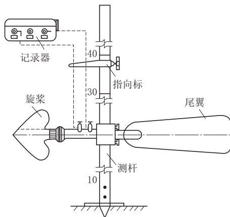
图 1.2 旋桨式流速仪
