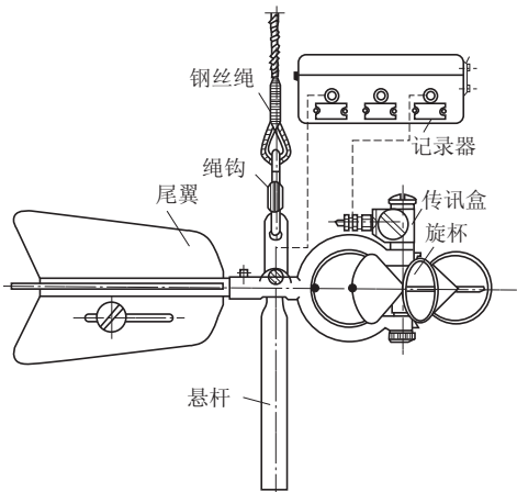
图 1.1 旋杯式流速仪
