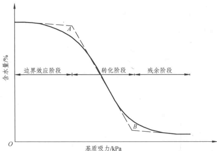
图 1.2-1 典型非饱和土水土特征曲线
