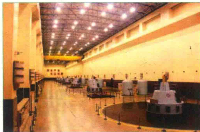
水口水电站发电厂房（摄于1996年）
