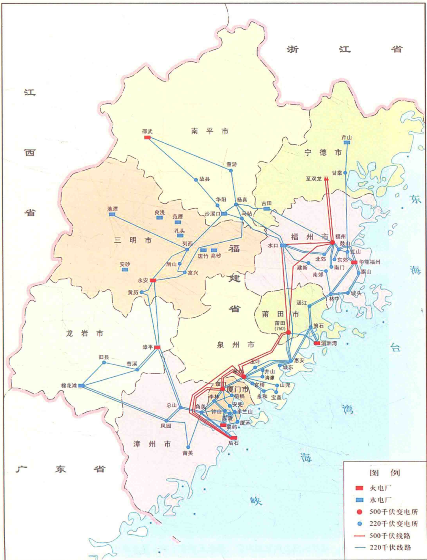
2002年福建省电网接线示意图
