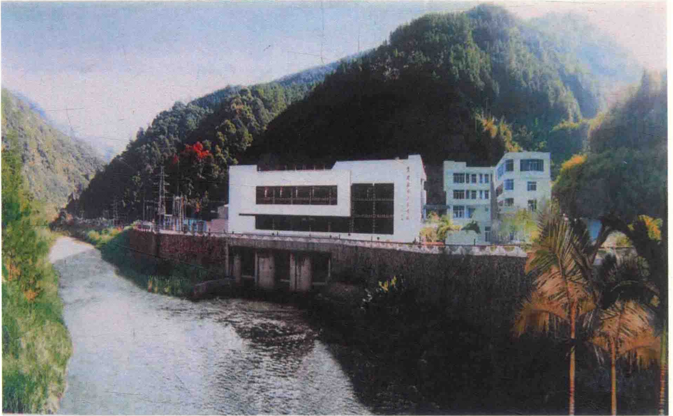
由福建省电力局、龙岩地区行政公署、龙岩市政府、国家能源中型水电实业开发公司、福建省中闽公司合资兴建的龙岩万安溪水电厂，装机3台总容量4.5万千瓦（摄于1994年）
