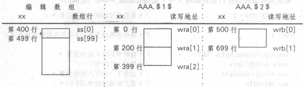
(1) 编辑数组后部 200 行移至临时文件 AAA.$2$
