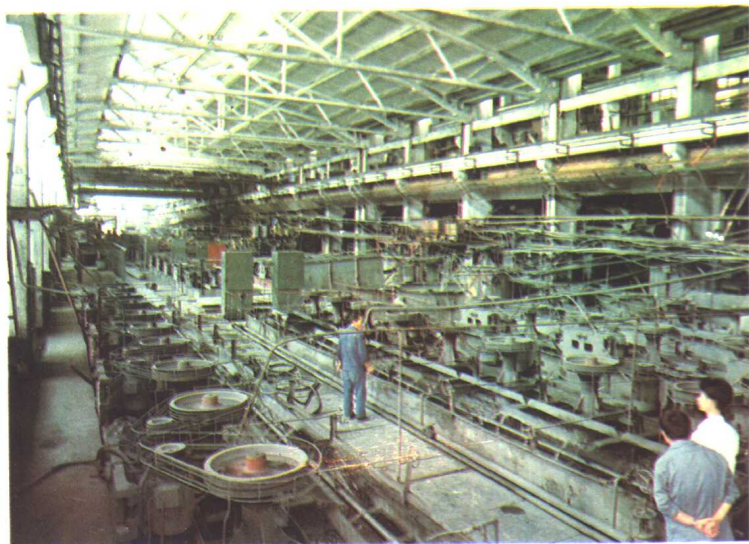
大厂矿务局车河选厂全浮系统。(王崇礼摄)
