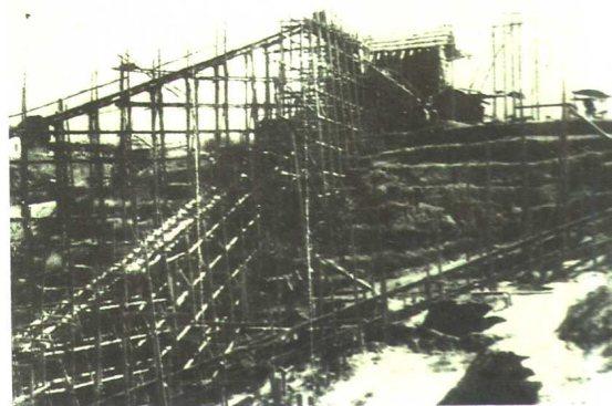
平桂矿务局20世纪20年代至60年代砂锡矿用的选矿设备木流槽——金沙沟。(平桂矿务局修志办供稿)
