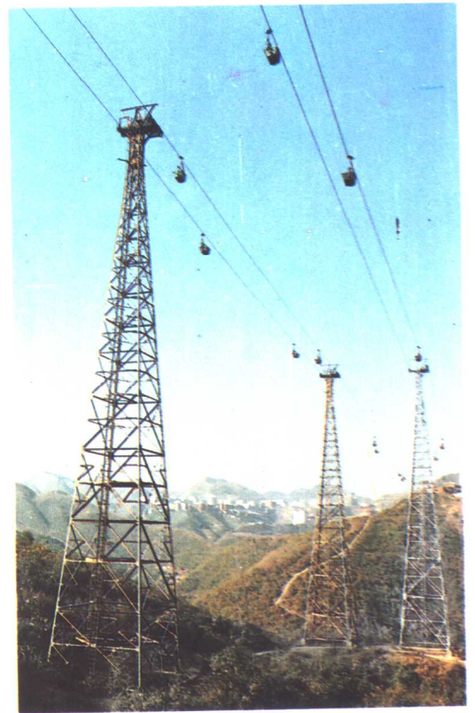
大厂矿务局铜坑至车河架空索道。(王崇礼摄)
