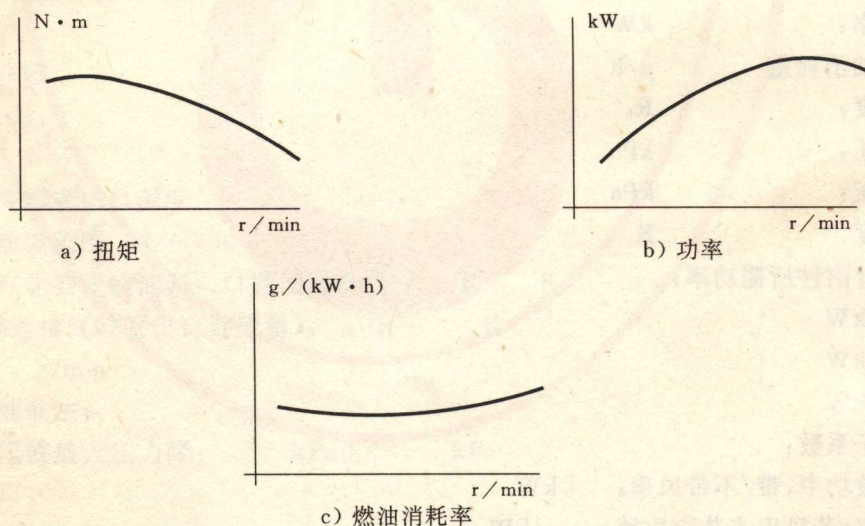
图 2 扭矩、功率和燃油消耗率的特性曲线
