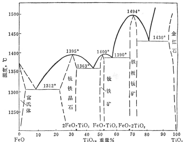
图 1-1 FeO-TiO 2 系状态图
