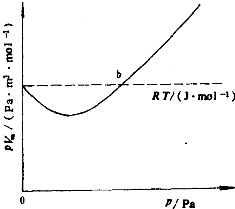
图 1.2.3 真实气体的 pV_m - p 图
