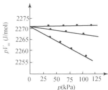
图 0-1 273.15K 下 Ne、O 2 、CO 2 的 pV_m-p 等温线
