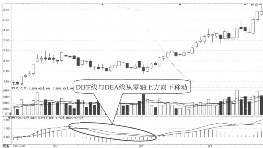
图 1-5 中国太保日 K 线
