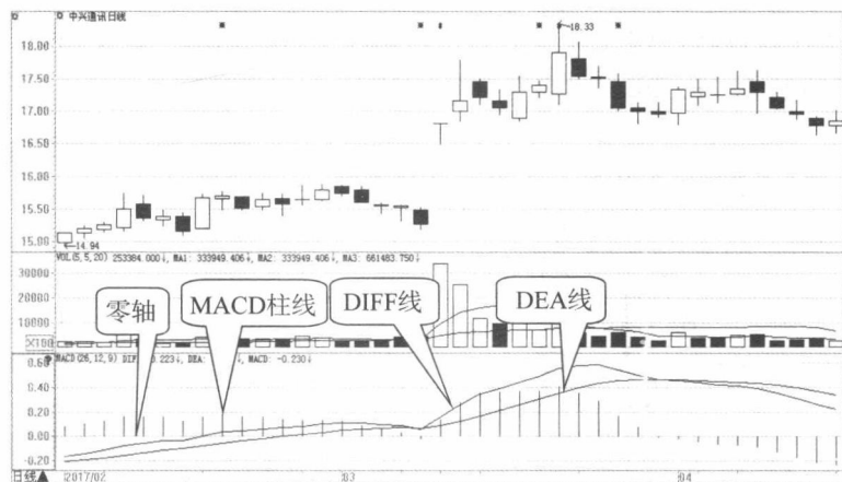
图 1-1 MACD 指标
