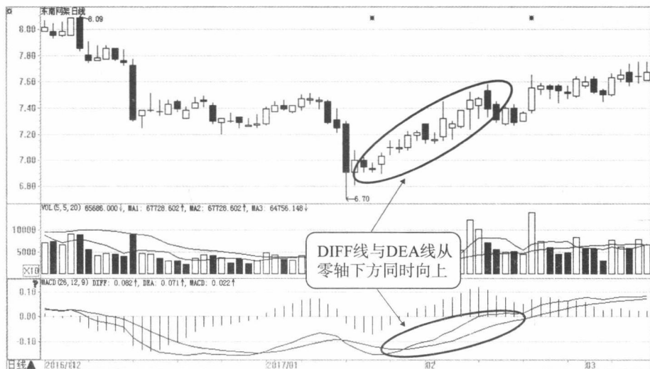
图 1-6 东南网架日 K 线
