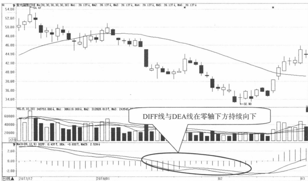
图 1-4 紫光国微日 K 线
