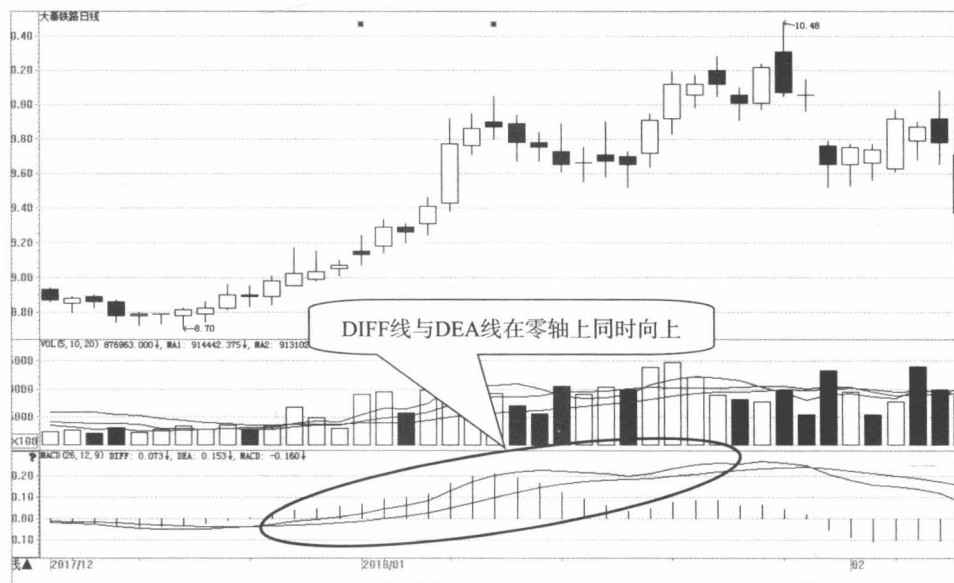
图 1-3 大秦铁路日 K 线
