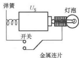
图 1-1 手电筒照明实际电路
