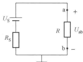
图 1-7 定义电压示意图
