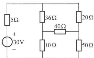
图 1-5 桥式电路
