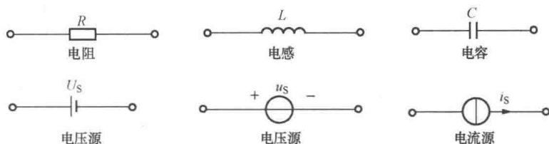
图 1-3 理想电路元件的图形符号
