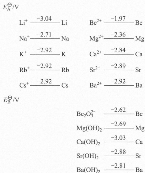
图 12-1 碱金属和碱土金属的元素电势图 ①
