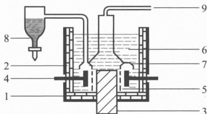
图 12-2 熔盐电解法生产钠的电解槽示意图
