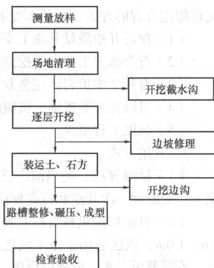
图1B411013 土质路堑施工工艺流程图
