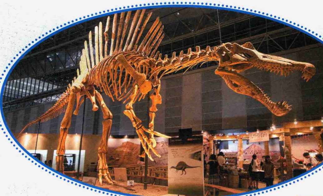
棘龙全身骨骼复原模型
