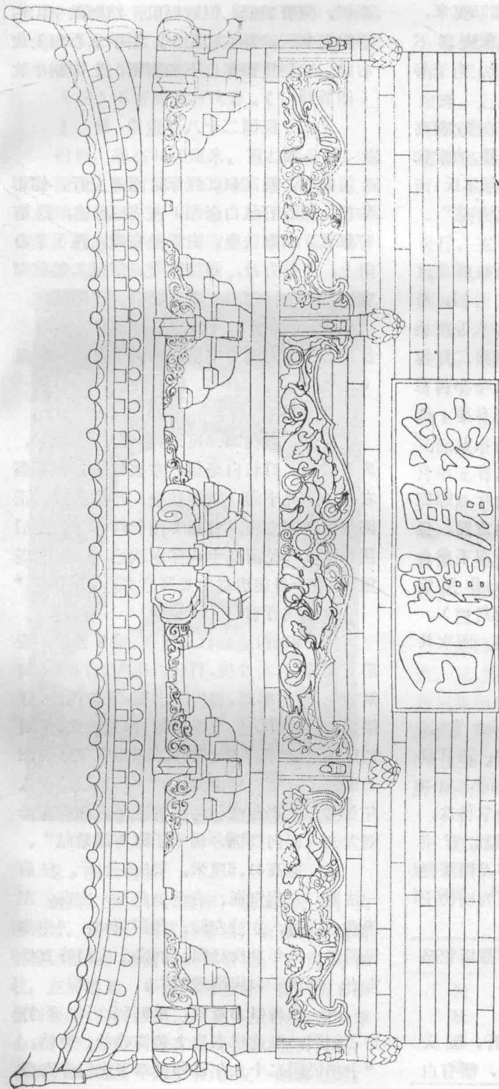
图三 法門寺東塔第一層細部立圖
