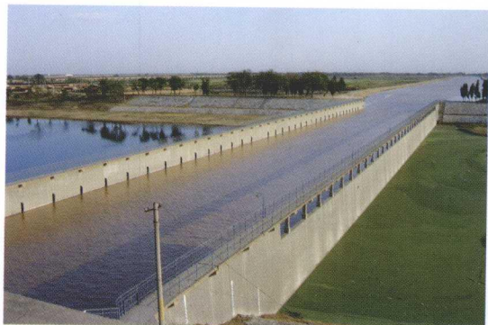
◆ 南运河穿运渡槽
