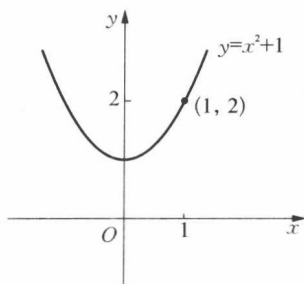
图 6.1 曲线 y = x^2 + 1 的图形
